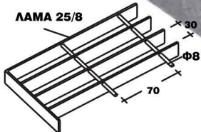
ΣΧΑΡΑ ΓΑΛΒΑΝΙΖΕ
