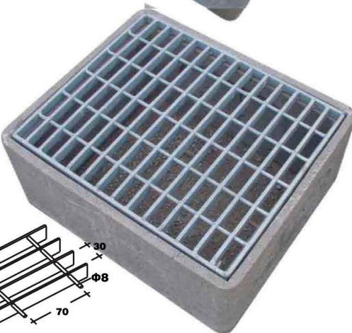
ΣΧΑΡΑ ΓΑΛΒΑΝΙΖΕ
