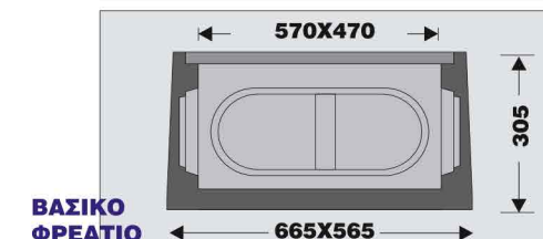
ΠΡΟΕΚΤΑΣΗ ΦΡΕΑΤΙΟΥ
