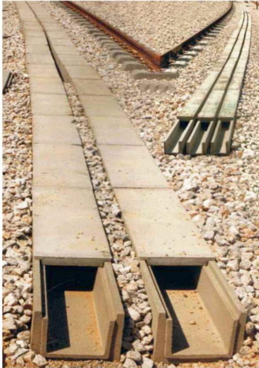
ΚΑΝΑΛΙΑ Κ160 & Κ90 ΤΟΠΟΘΕΤΗΜΕΝΟ ΣΤΟ ΑΤΤΙΚΟ ΜΕΤΡΟ
